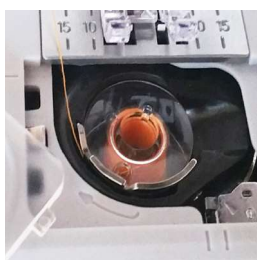
Crochet rotativo a carica dall'alto
